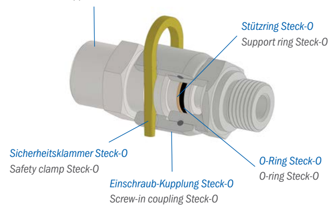
Aufschraub-Stecknippel Steck-O Screw-on nipple Steck-O
