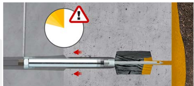
Injektionsrohr innerhalb der Verarbeitungszeit des Injektionsmaterials entfernen. | Remove the injection tube within the processing time of the injection material.
