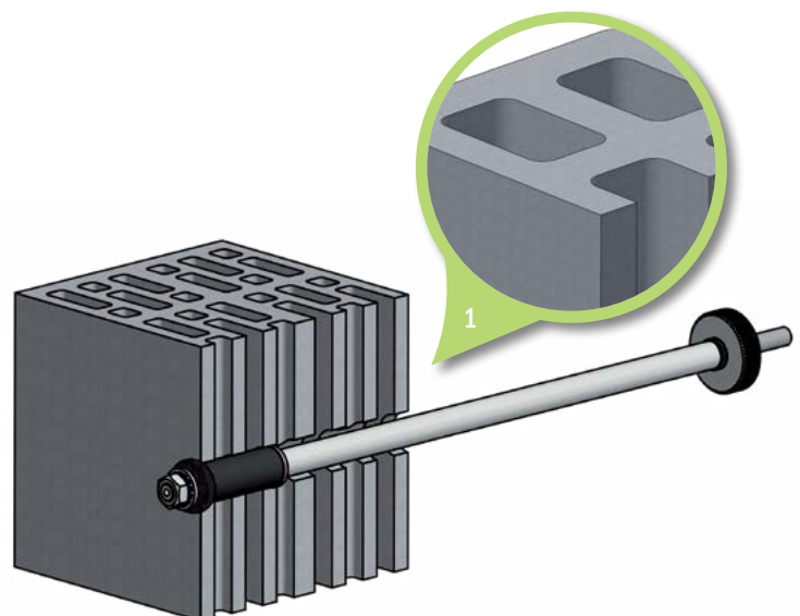
Injektionspacker gespannt im Lochziegelstein und Hohlblockstein (1) Injection packer clamped in the perforated brick and cavity block (1)
