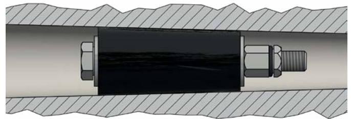
TW-Blindpacker gespannt im konischen Bohrloch TW blind packer clamped in conical borehole
