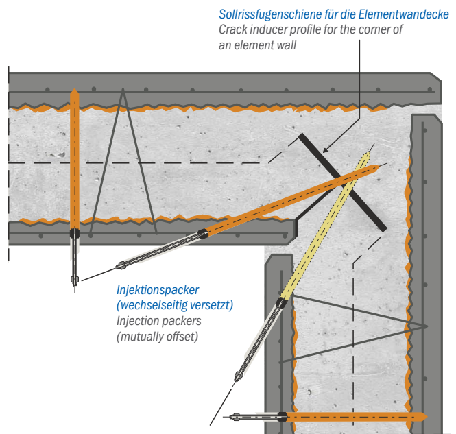
Nachträgliche Abdichtung einer Elementwandecke mit einer Sollrissfugenschiene Subsequent sealing of an element wall corner with a crack inducer profile
