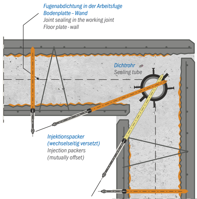
Nachträgliche Abdichtung einer Elementwandecke mit Dichtrohr durch Injektion Subsequent sealing of an element wall corner with sealing tube by injection
