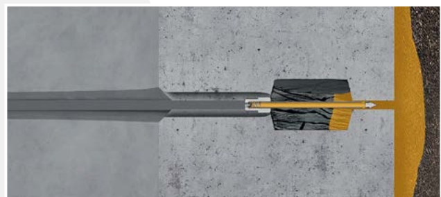
Abgeschlossene Injektion, B-STING® Fugeninjektionsnadel verbleibt in der Dichtung
