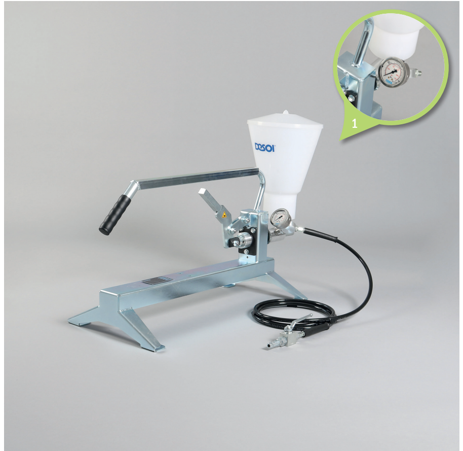
1. Manometerkombination
